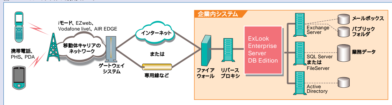
図1 ExLookのシステム構成イメージ
